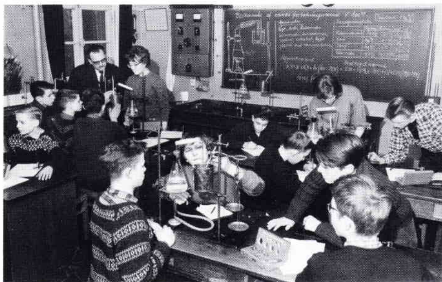
Billedet viser Lindersdorf i lokalet på Sjællandsgades Skole (engang i 50'erne) i gang med elevovvelser. Det er en af de yndede kalorimeterøvelser (fordampnings-/fortætningsvarme). Til venstre for tavlen ses spændingsforsyningen, en dynamo (0-20 v DC, max. 20 amp.) til lærer- og elevforsyning. Under den en kasse med lærerens vekselspænding (22 v AC uregulerbar). Elevborde havde ikke vekselspænding.
