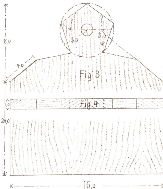
Skærebræt 7 A. Fig. 3-4.
