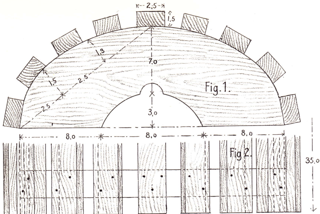
Havaskammel 5 A. Fig. 1—8.
