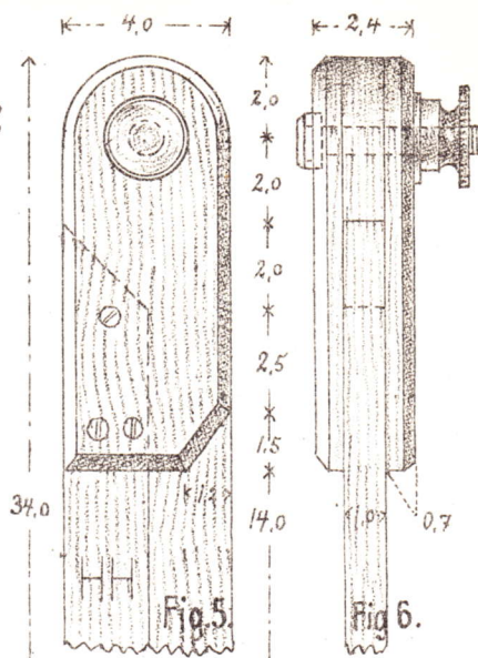
Kridtpasser 7 C. Fig. 5—7.
