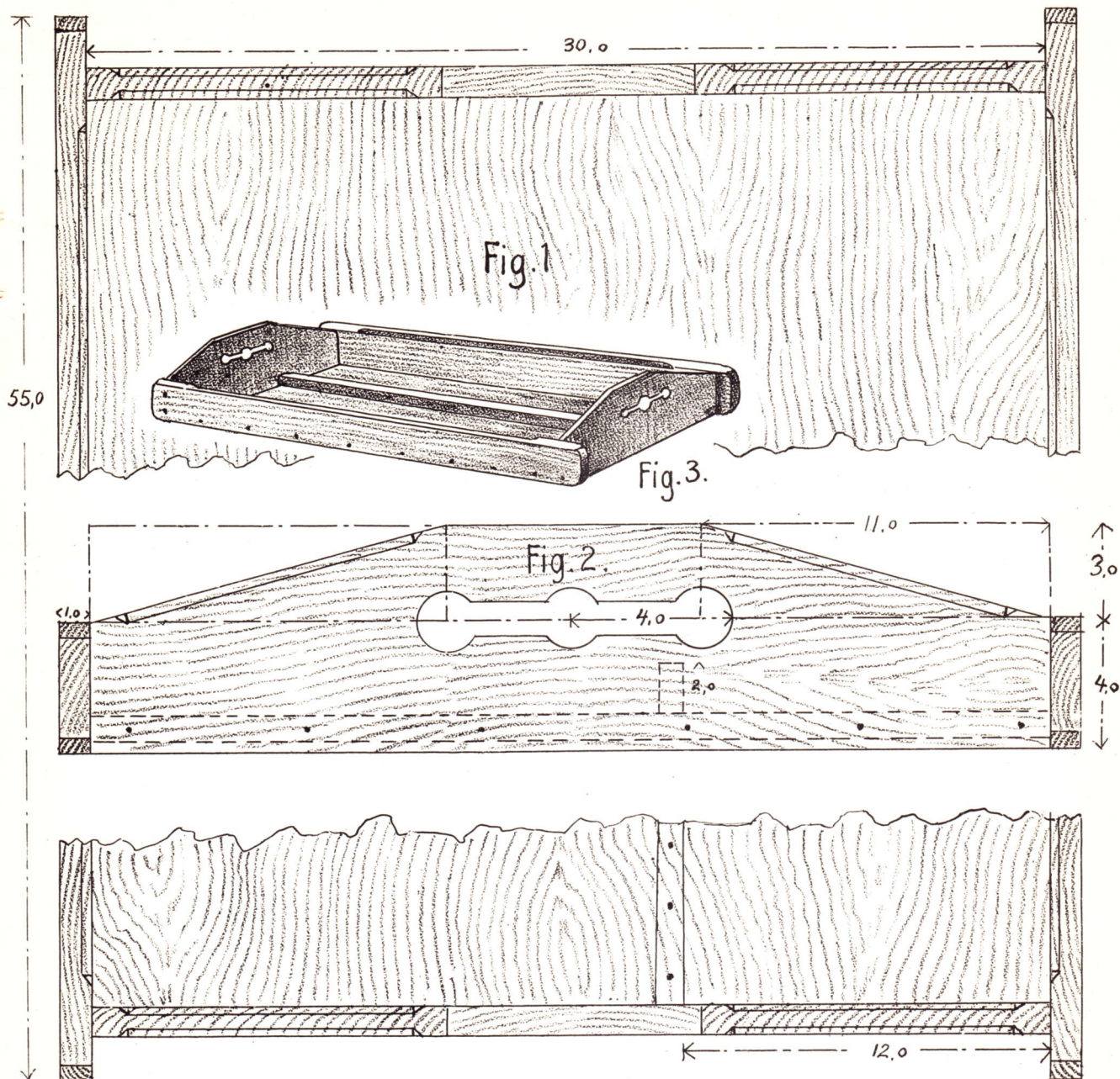
Tallerkenbakke 3 F. Fig. 1—3.
