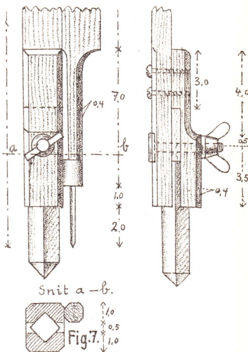
Nøglebræt 7 C. Fig. 3—4.
