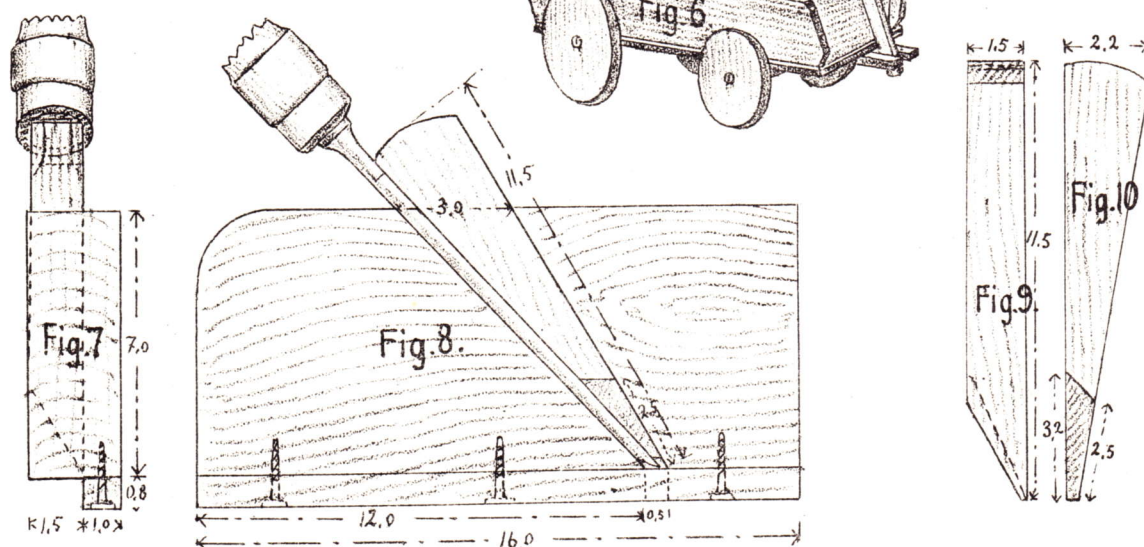
Falshevl 6 B. Fig. 7—10.
