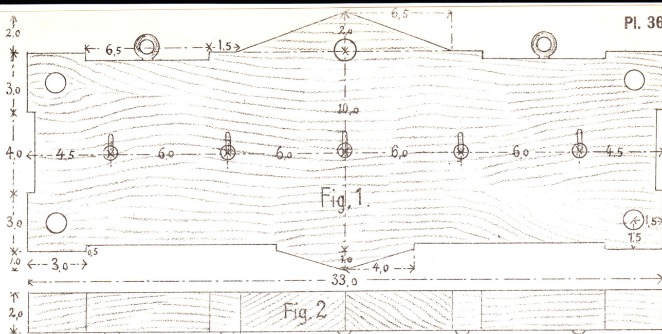
Pibebræt 7 A. Fig. 1-2.
